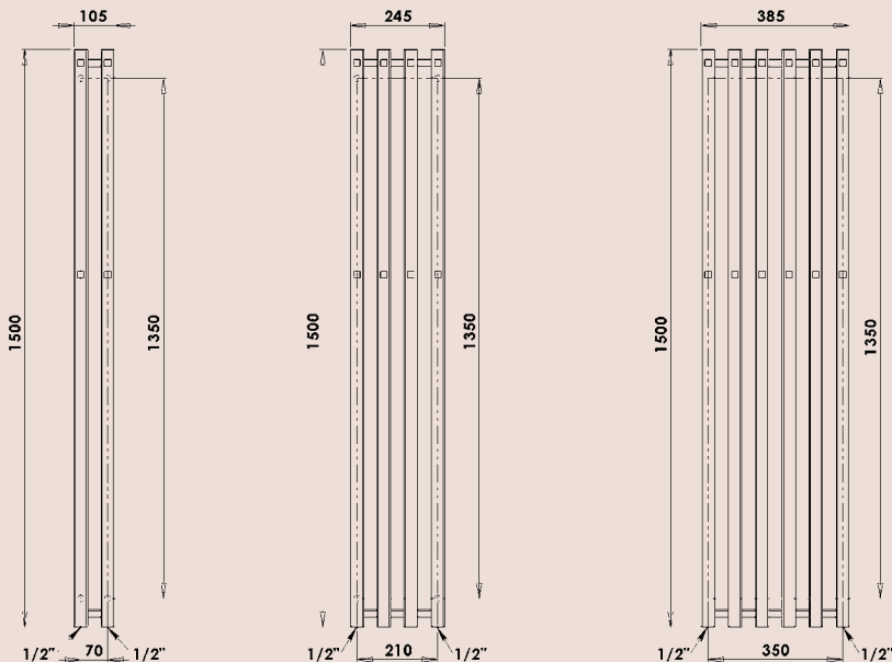
PLUTO P2C/6 – vyhotovenie chróm 385 × 1500 mm
